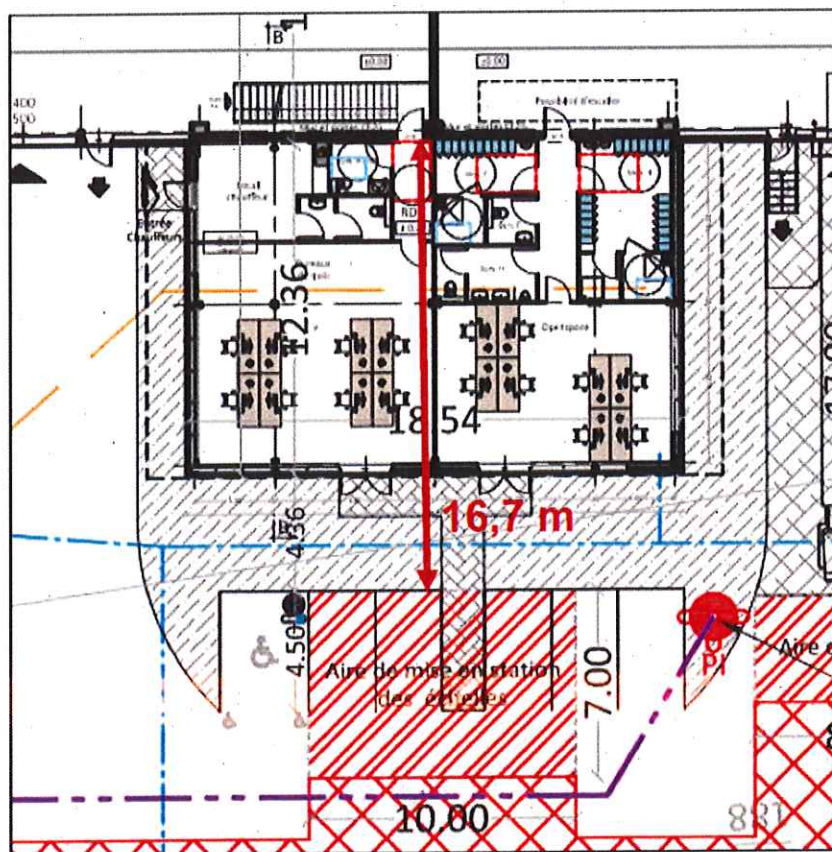
Extrait plan : distance aire/mur inter-cellule
